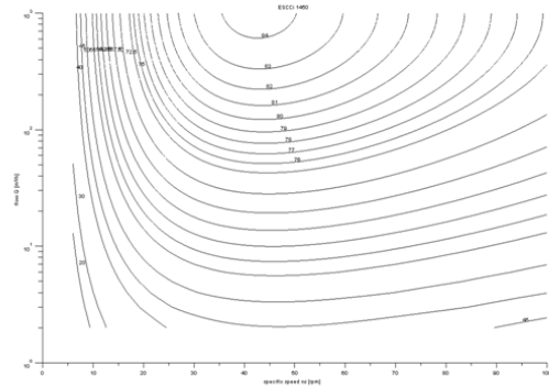
Przykład wykresu sprawności wzorcowej
