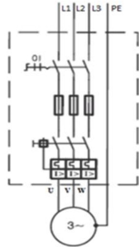
Rys. 1 Schemat elekt. Podłączenia pomp 3-fazowych
