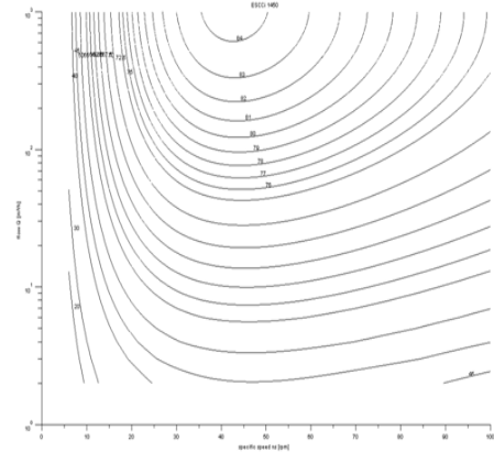
Przykład wykresu sprawności wzorcowej
