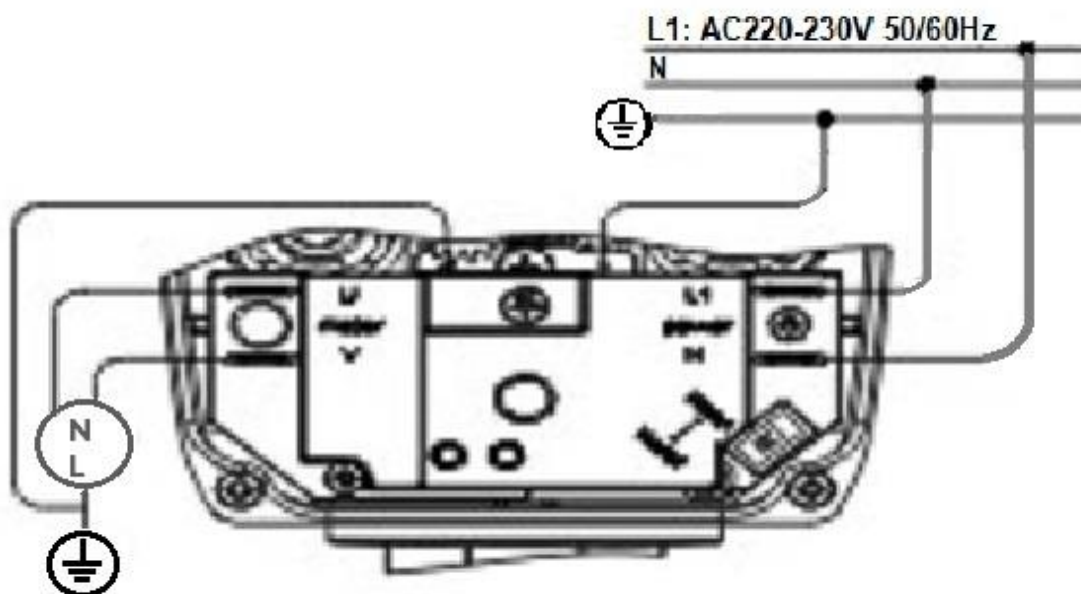
Schemat podłączenia Automatycznego Sterownika Ciśnieniowego OPC-59 z jednofazową pompą o mocy do 1,1 kW
