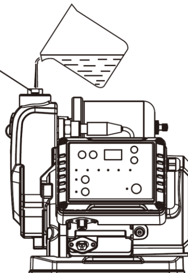
Rys. 3 Zalewanie pompy
