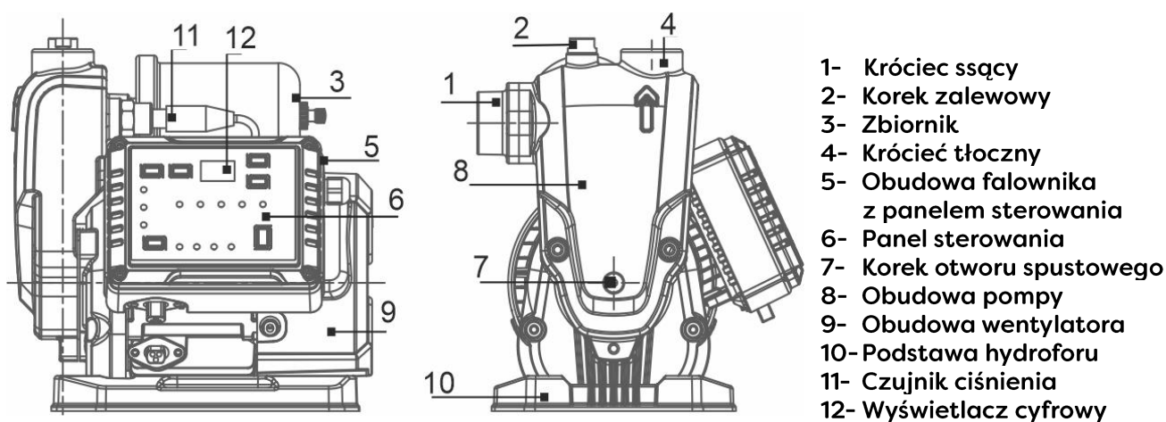
Rys. 1 WZ 900 SMART/WZ 1500 SMART
