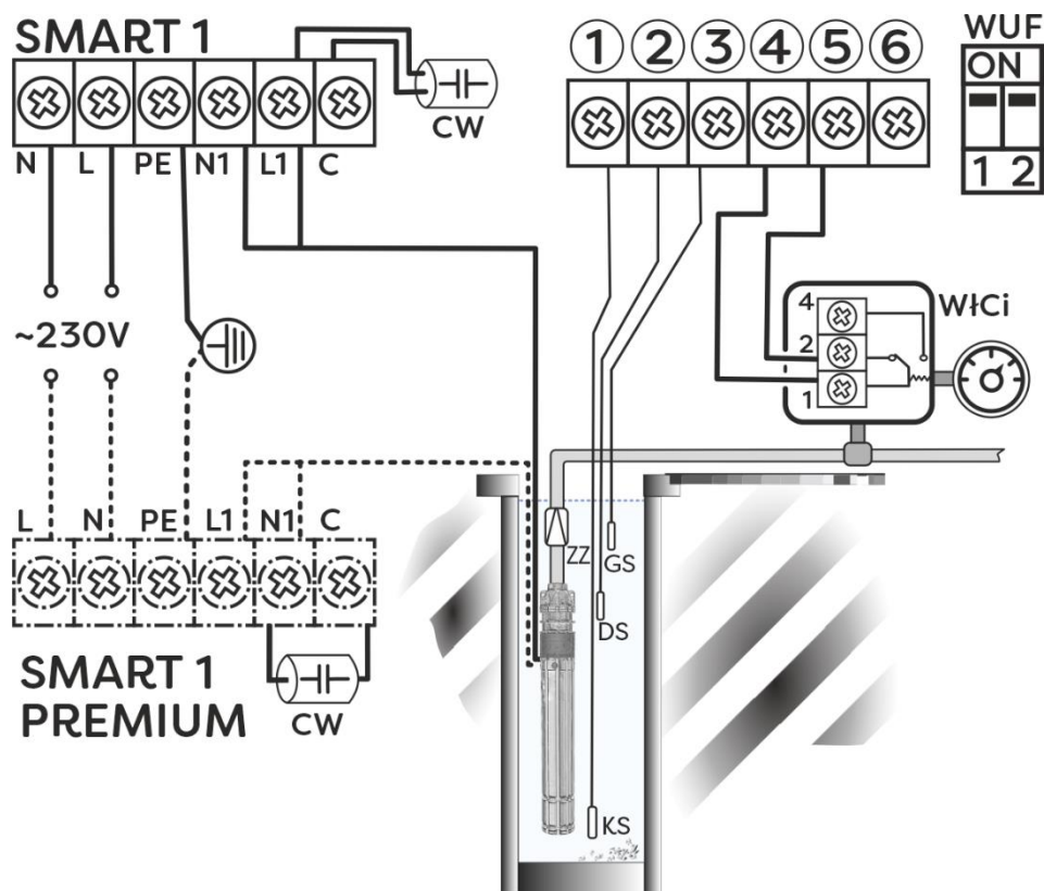
Schemat 6. Silnik pompy 230 V (z wbudowanym w nim kondensatorem rozruchowym) sterowany ciśnieniem w instalacji tłocznej za pomocą włącznika ciśnieniowego i zabezpieczony poprzez kontrolę poziomu wody sondami
