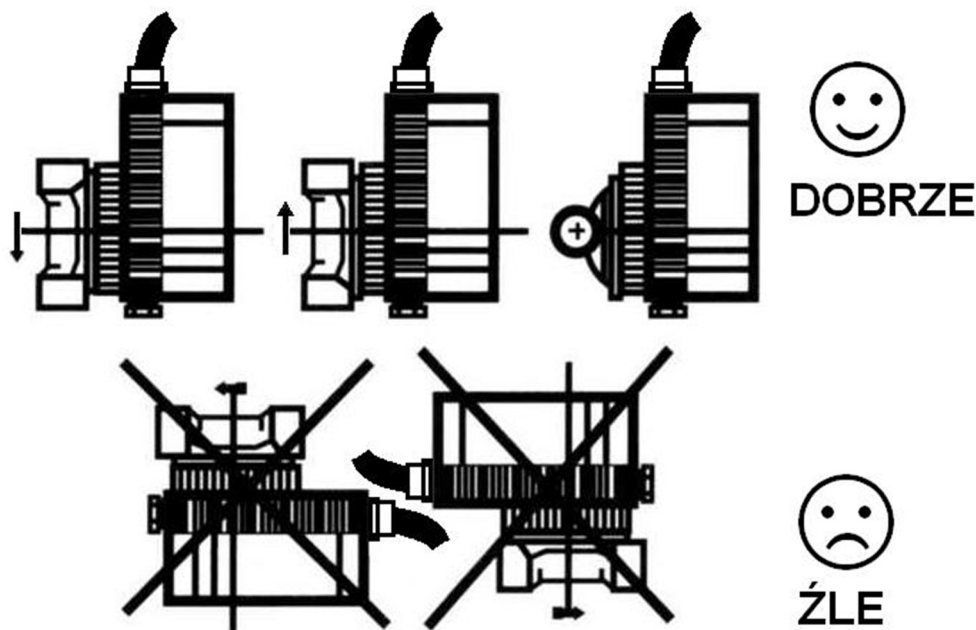
Rys. 3 Sposób montażu
