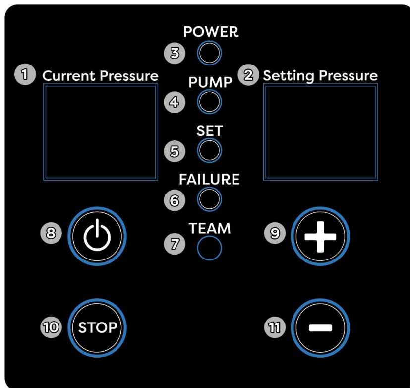
Rys. 2 Opis rozmieszczenia przycisków i komunikatów
