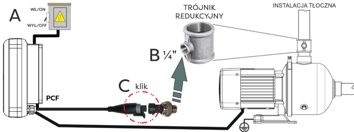
Rys.11 Przykładowe podłączenie czujnika do instalacji tłocznej
